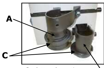
Goulottes de sortie: A Pièces Comptées B Pièces rejetées (Tri) C Fixations rapide des sacs
